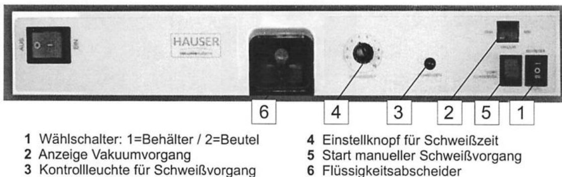
Abbildung 2: Steuerungen Hauser 550
